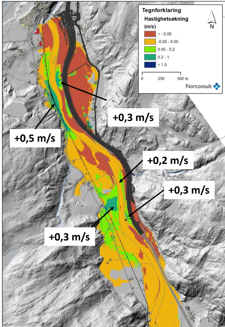
Figur 3-13: Alternativ 1.1.C Gyllan – Hovin. Hastighetsøkning etter tiltak, maksimale hastigheter under flomforløp 1,2 x Q200 i Gaula (Kilde: Norconsult).
