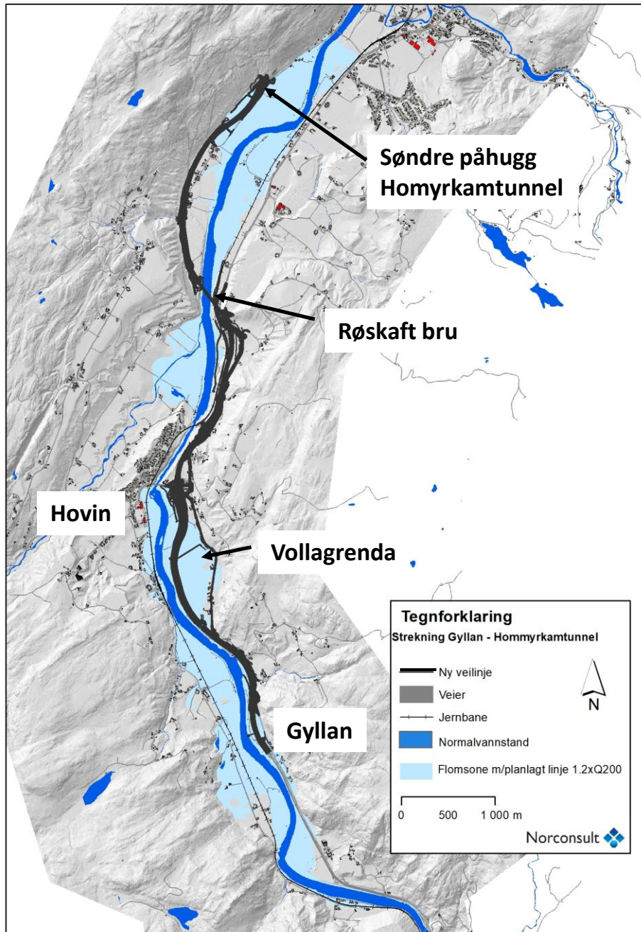
Figur 3-3: Oversikt strekning Gyllan - Homyrkamtunnel og flomutsatt område ved Q200 + 20 % klimapåslag (Kilde: Norconsult).
