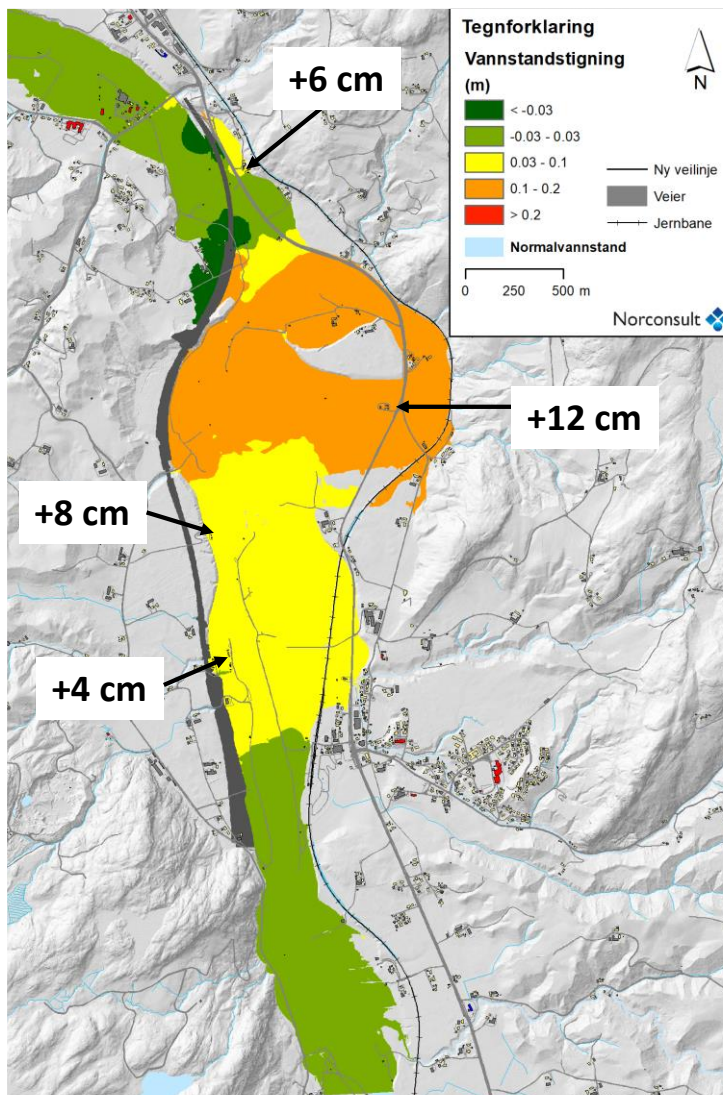
Figur 4-6: Alternativ 2.1. Vannstandstigning med planlagt E6 og Kåsabrua (Kilde: Norconsult).
