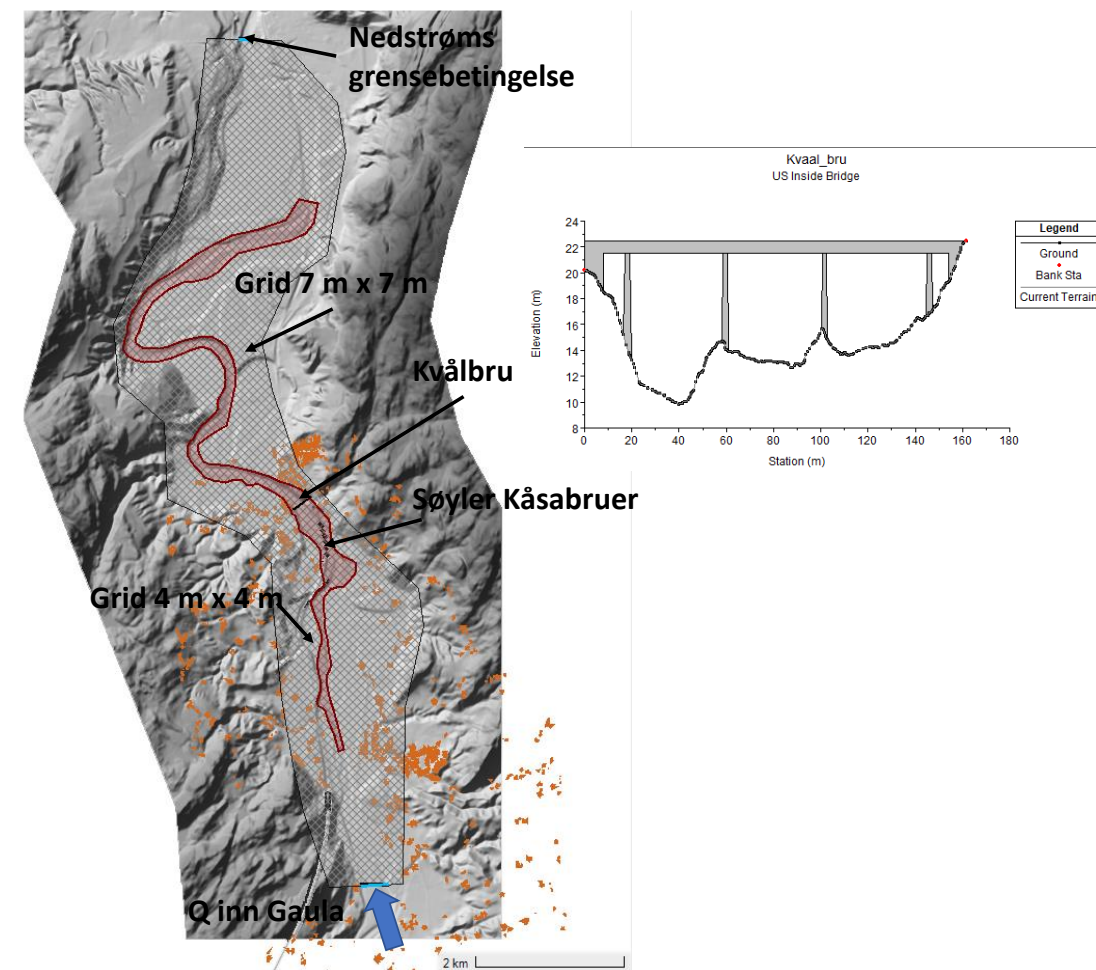
Figur 4-3: Alternativ 2.1. 2D-modell i Hec-Ras (Kilde: Norconsult).
