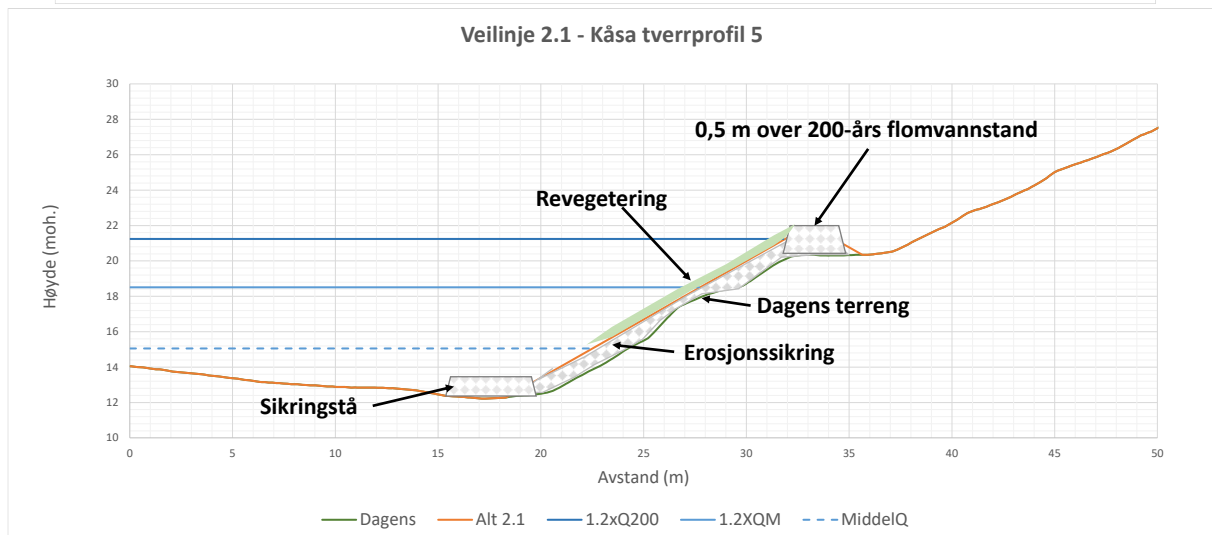
Figur 5-12: Prinsippskisse for erosjonssikring i Gaula ved Kåsa, erosjonssikring ved Kåsa er lagt over eksisterende terrengnivå (sett fra sør mot nord) (Kilde: Norconsult).
