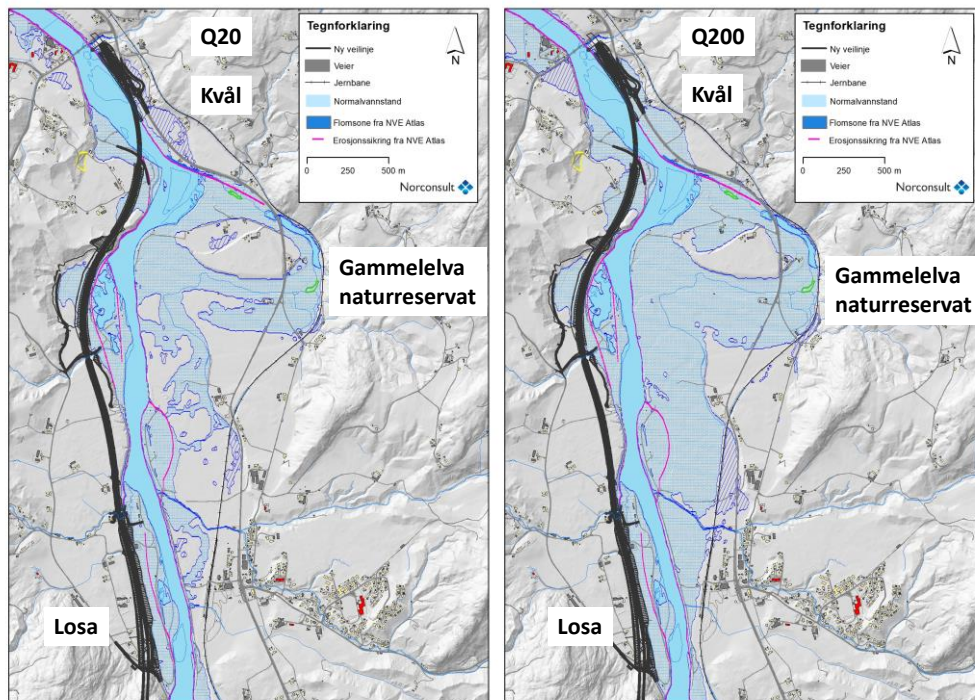
Figur 2-4: Flomutsatt område på strekning Homyrkamtunnel nord/ Løsa og Kvål ved Q20 og Q200 (Kilde: flomsone og eksisterende erosjonssikringstiltakene er hentet fra NVEs database [4]).
