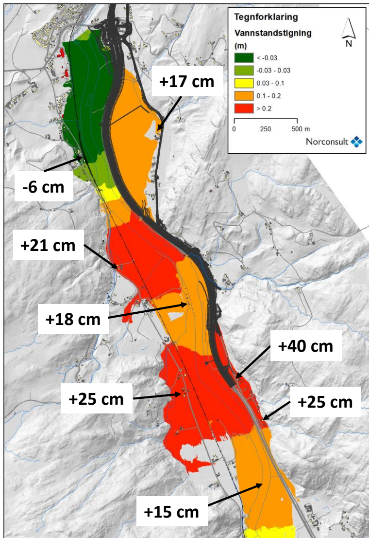
Figur 3-8: Alternativ 1.1.C Gyllan – Hovin. Vannstandstigning etter tiltak, flomsituasjon er kulminasjon av flomforløp 1,2 x Q200 i Gaula (Kilde: Norconsult).
