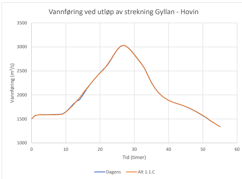
Figur 3-4: Vannføring ved utløp av strekning Gyllan – Hovin, dagens situasjon og med veilinje alternativ 1.1C.
