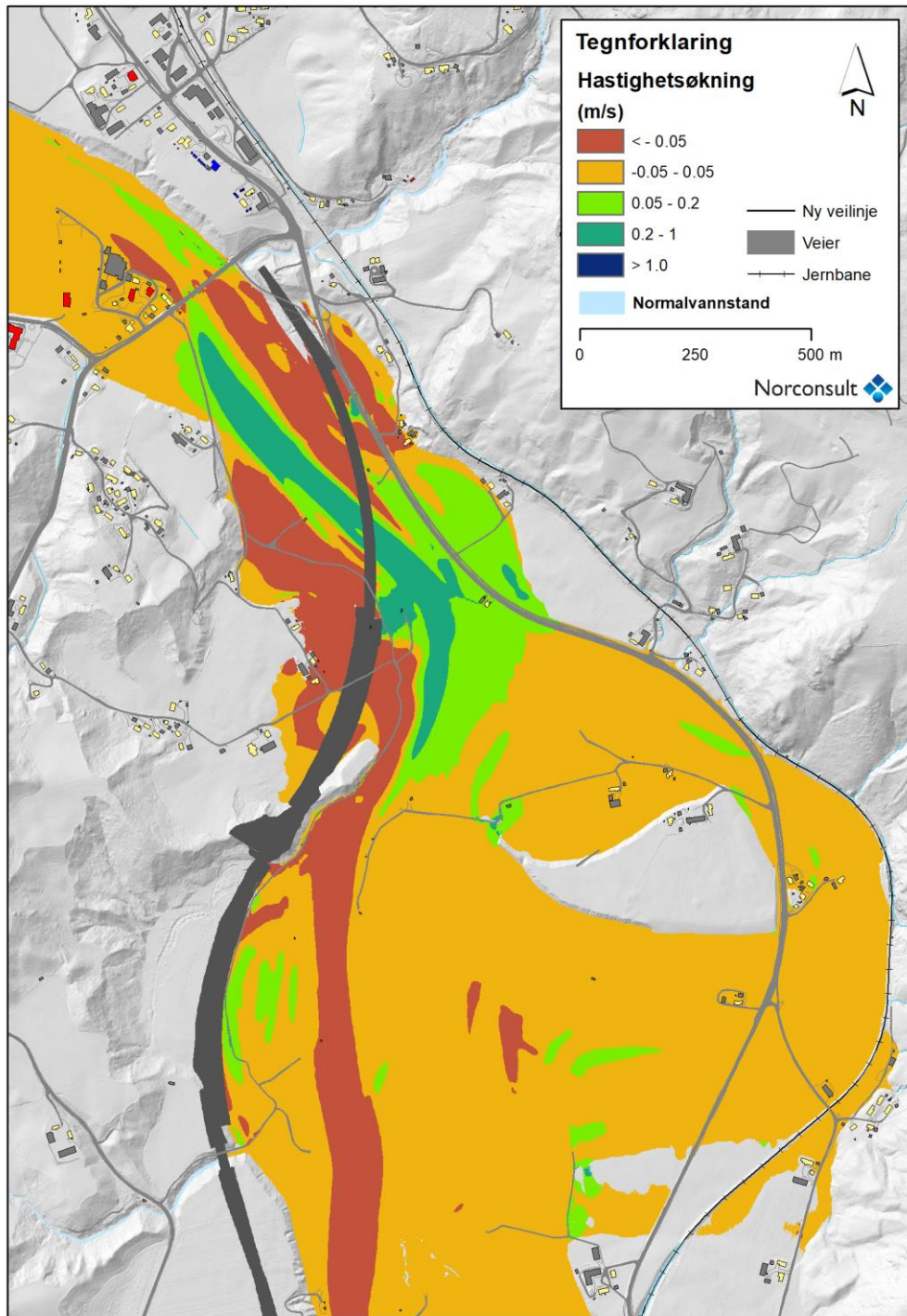
Figur 4-9: Alternativ 2.1 detalj Kåsabrua. Hastighetsøkning etter tiltak, flomsituasjon kulminasjon av flomforløp 1,2 x Q200 i Gaula (Kilde: Norconsult).
