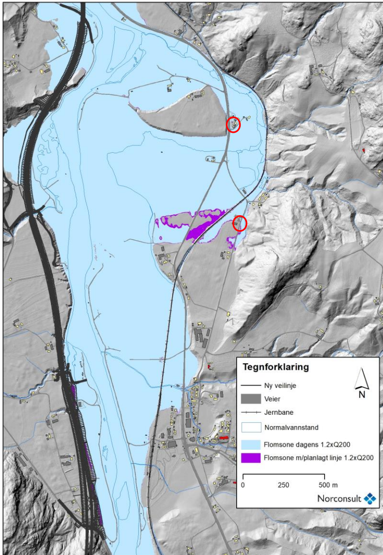
Figur 4-5 Losa - Kvål. Økning i flomutsatt område som følge av tiltaket (kilde: Norconsult).
