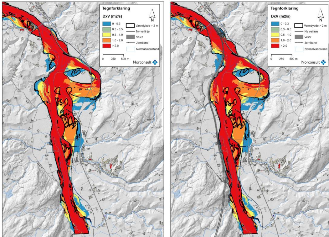
Figur 4-11 Losa - Kvål. Faregrad for flomutsatte områder, dagens situasjon (til venstre) og etter tiltak (til høyre) (Kilde: Norconsult).
