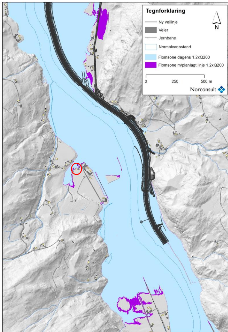
Figur 3-6 Gyllan – Hovin. Økning i flomutsatt område som følge av tiltaket (kilde: Norconsult).
