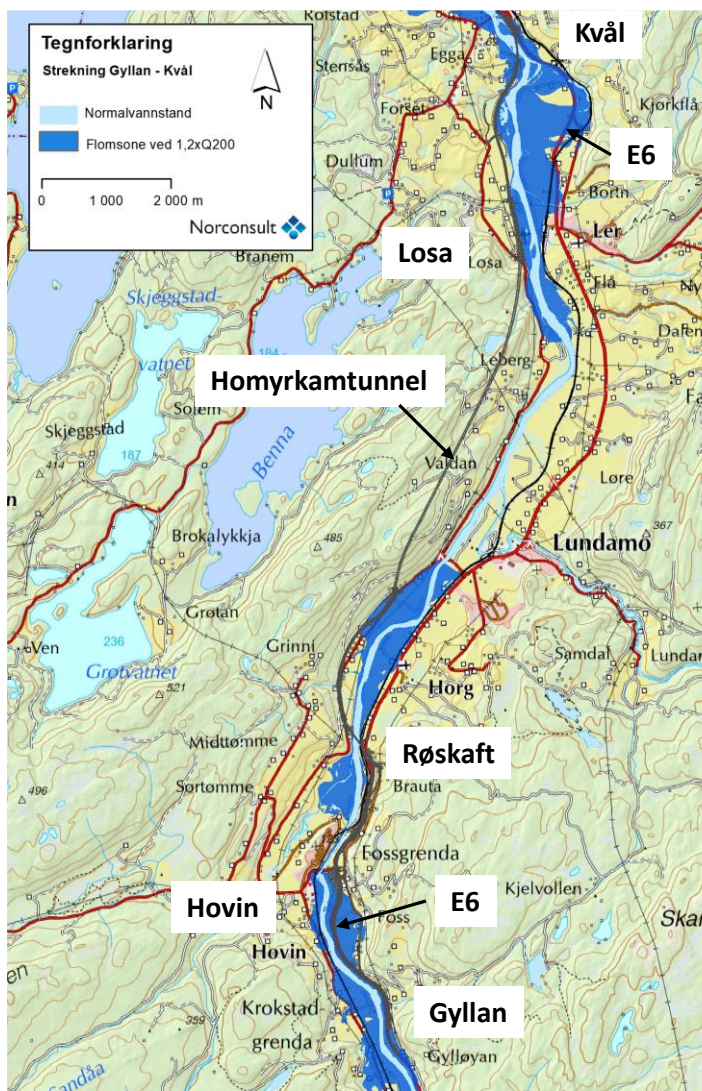
Figur 2-1 Oversikt over den planlagte linje mellom Gyllan og Kvål og flomutsatt område ved 1,2xQ200. E6 går i dag på østre siden av Gaula, og er vist i rød farge. Flomsone i Gaula der ny E6 er planlagt i tunnel er ikke beregnet (Kilde: Norconsult).
