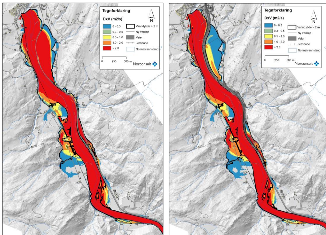
Figur 3-16 Gyllan – Hovin. Faregrad for flomutsatte områder, dagens situasjon (til venstre) og etter tiltak (til høyre) (Kilde: Norconsult).
