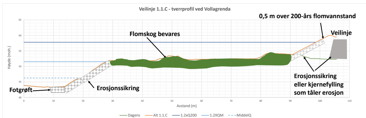
Figur 5-8: Prinsippskisse for erosjonssikring i Gaula, stor avstand mellom veilinjen og Gaula, området dekket av flomskog (Kilde: Norconsult).
